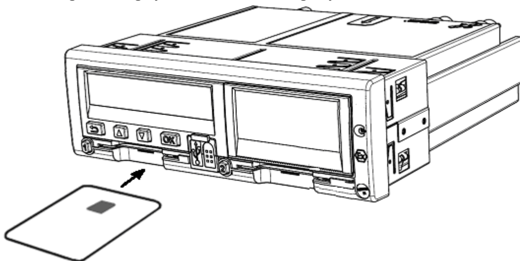
Рисунок 3 – Установка карты водителя в картоприемник «Основной водитель»
